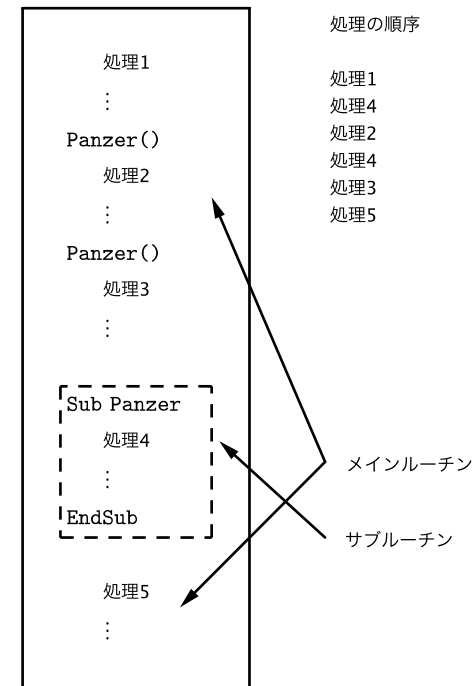
図 14: サブルーチンの処理の順序
