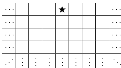
図 16: 3 方向に無数のマスのある盤面
