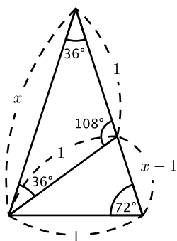
図 18: 黄金比の現れる三角比
