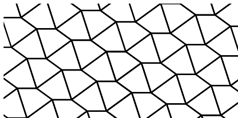
図 46: カイトによる違法なタイリング
