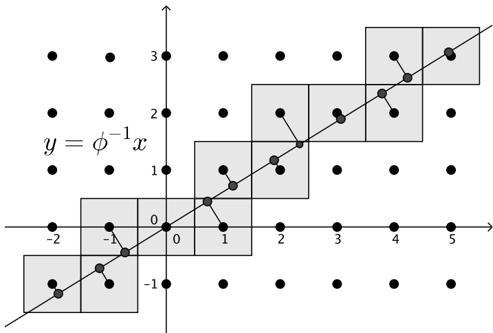
図 65: 正射影
