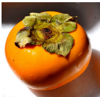
図 26: カキ
