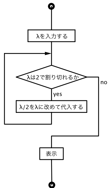
図 9: 課題 17 の流れ図
