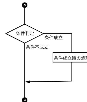
図 5: If 文の流れ図
