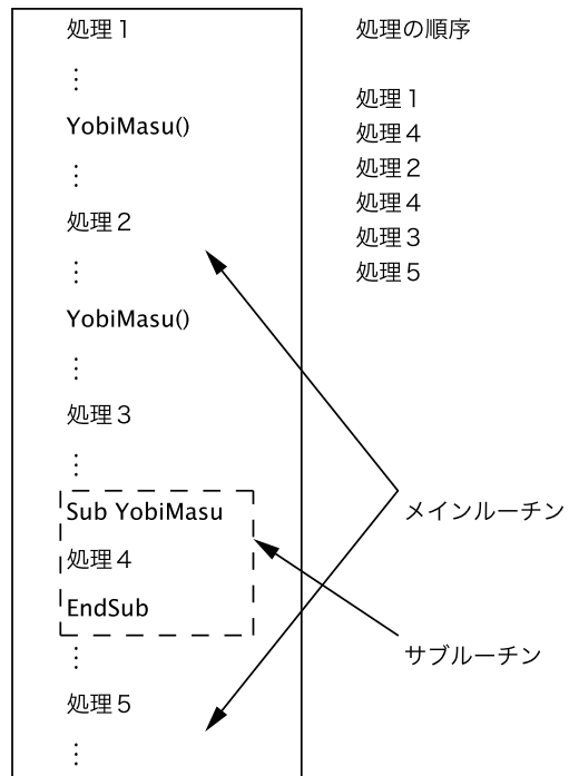
図 10: サブルーチンの処理の順序
